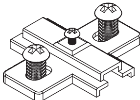
Hinge Plate with screws (4) Plaque de charnière avec les vis RM-0018
