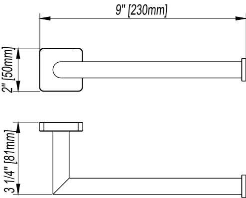
ROLL HOLDER / PORTARROLLOS / PORTE-ROULEAU
