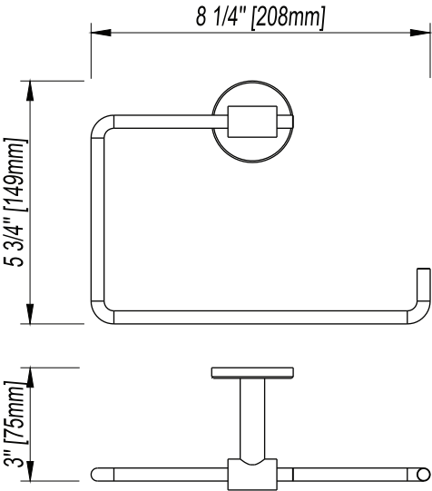
ROLL HOLDER / PORTARROLLOS / PORTE-ROULEAU
