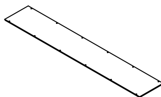
Top panel - slide / Panneau supérieur - coulissant (1pc)
