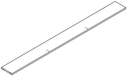
⑤ 1600*150*15= 1PCS
