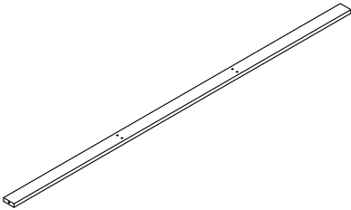
⑥ 1600*50*15= 1PCS
