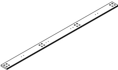
⑪ 1583.5*86*15= 1PCS
