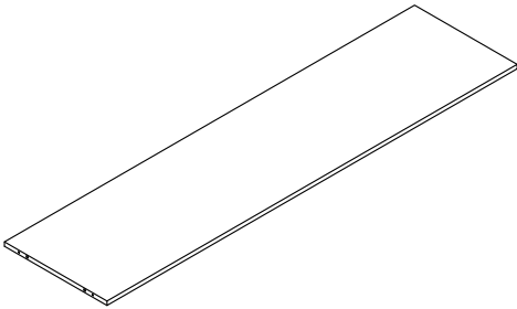
⑨ 1600*400*15= 1PCS
