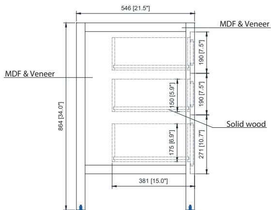
Side / Côté
