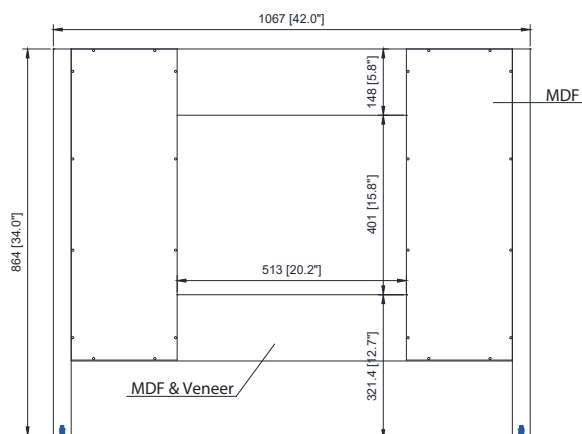
Back / Derrière
