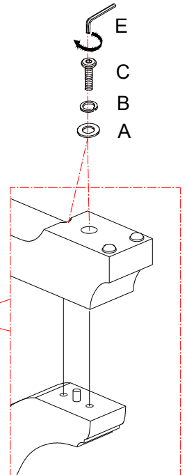
Step/ Étape/ Paso 3
