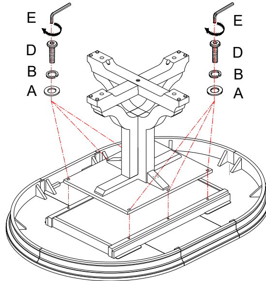
Step/ Étape/ Paso 7
