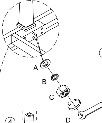
Step/ Étape/ Paso 2
