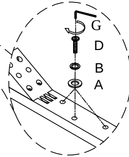
Step/ Étape/ Paso 2
