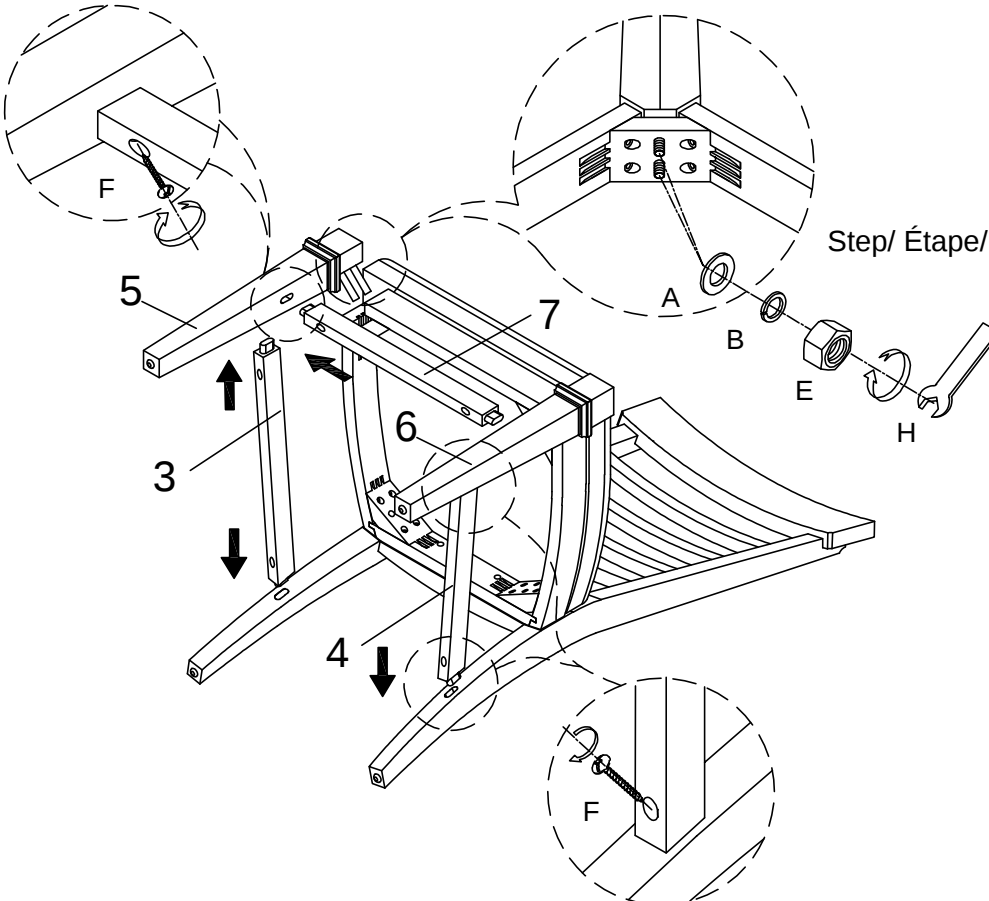
Step/ Étape/ Paso 5
