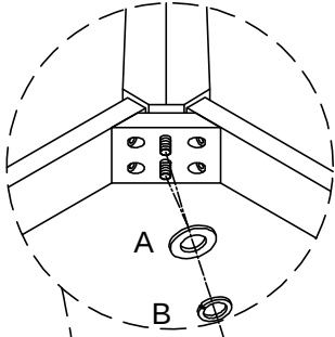
Step/ Étape/ Paso 1
