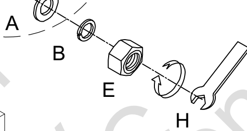
Step/ Étape/ Paso 4
