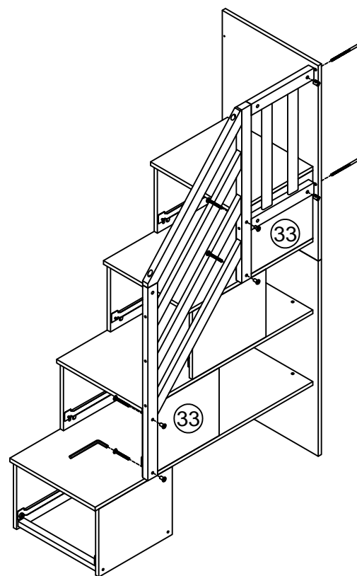
Ladder on right side Échelle du côté droit
