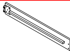
Side rails - 2pcs Rails latéraux - 2pièces
