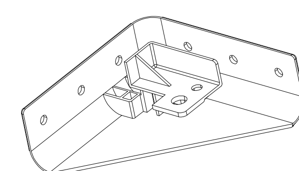
F35-C28 x1
