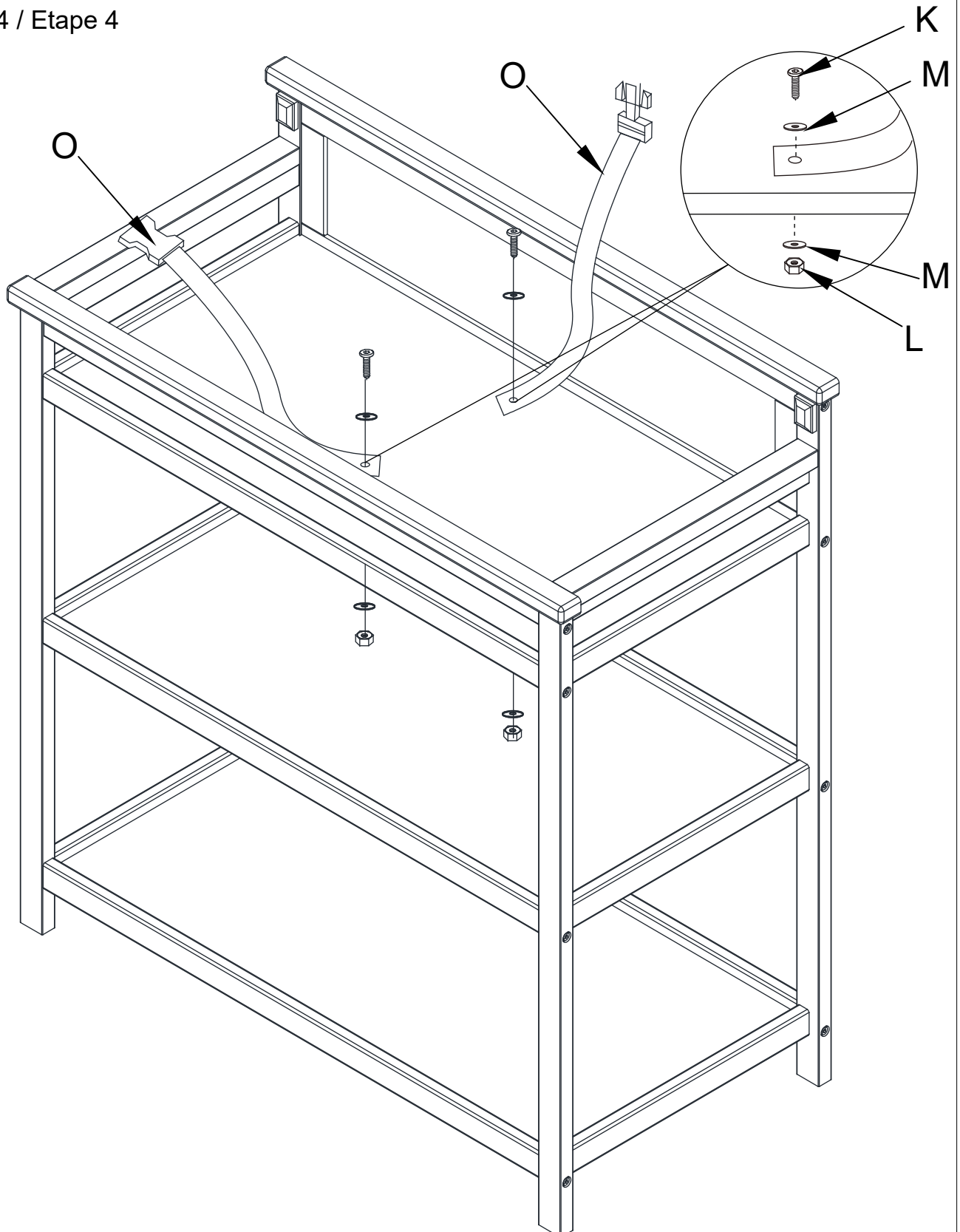
(M) Metal Washer / Rondelle métallique ( x 4 )
