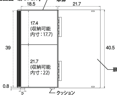
[正面図・扉OPEN]
