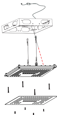
Stainless steel fix frame Cadre de fixation en acier inoxydable
