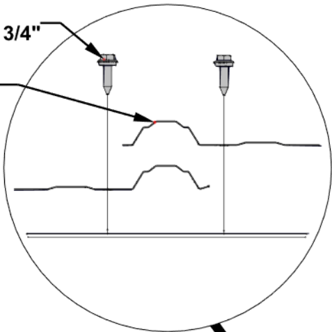
A4M02639 (x2) 29 GA STEEL SHEETING
