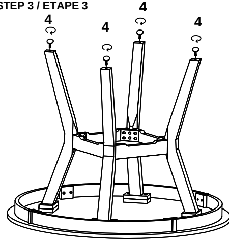
STEP 3 / ETAPE 3
