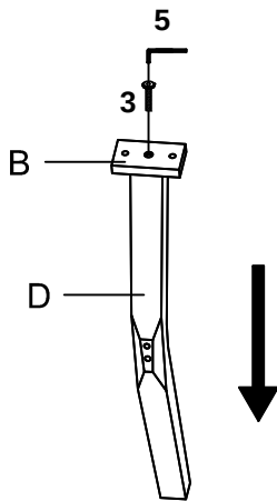
STEP 1 / ETAPE 1
