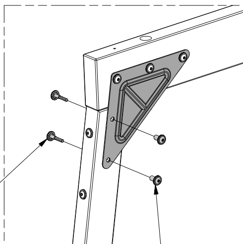
005 (x2) NUT BARREL - 7/8"
